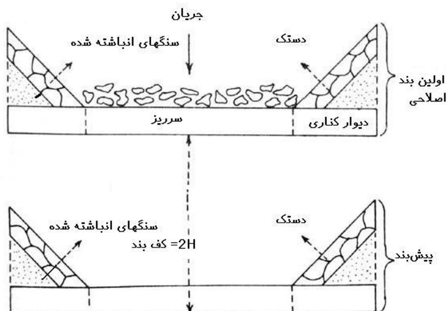
شکل شماره ۱۱- تصویر اولین بند اصلاحی خشکچین همراه با پیش بند (Geyik، ۱۹۸۶)
