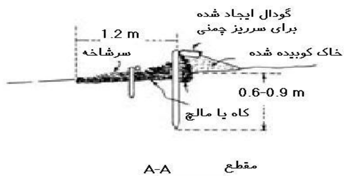
شکل شماره ۲- مشخصات بندهای فلزی سبک
