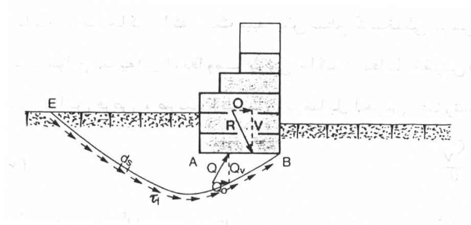
شکل شماره ۴۱- سطح گسیختگی برشی در پی سرریز توریستی (جوان و همکاران، ۱۳۶۹)
