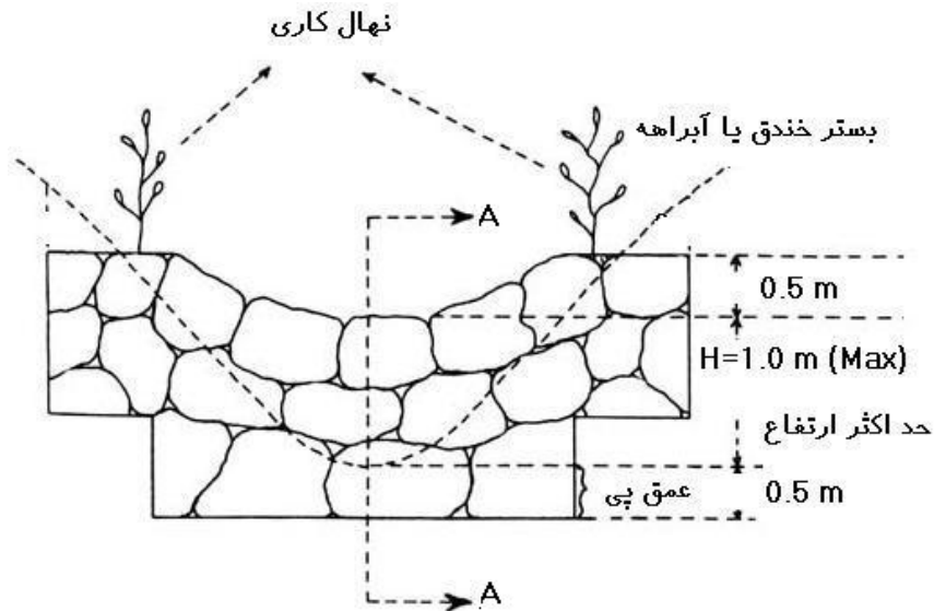
شکل شماره ۹- نمای جلوی بند اصلاحی خشکه‌چین (Geyik ، ۱۹۸۶)
