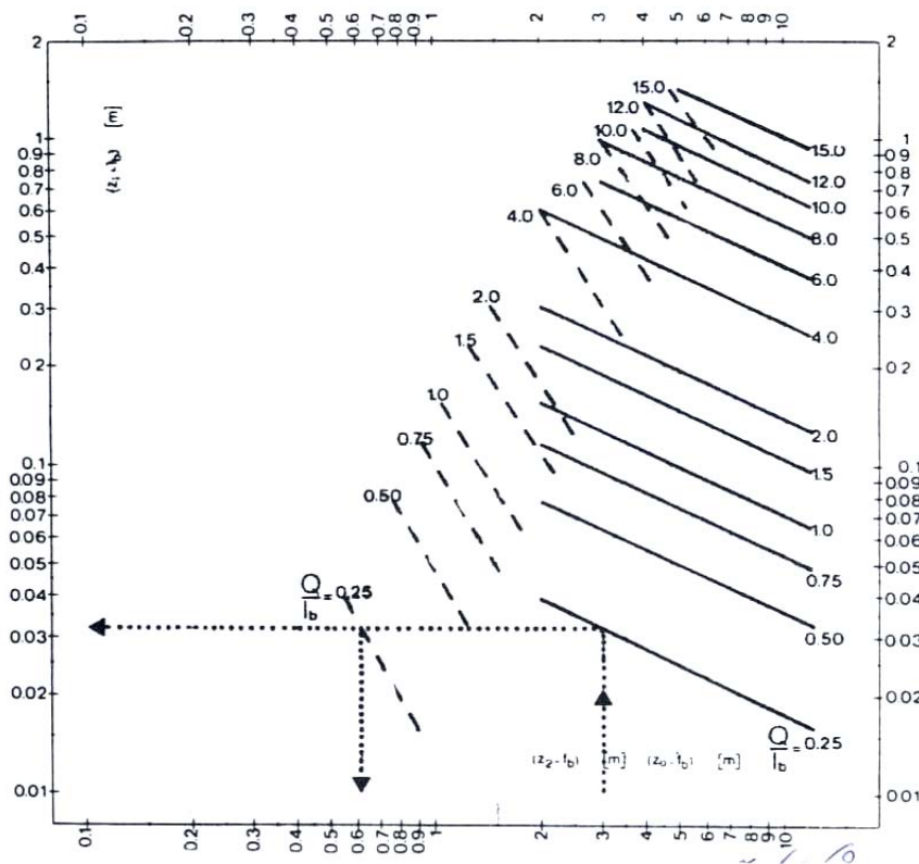
شکل ۳۶: نمودار تغییرات دبی سرریز (جوان و همکاران، ۱۳۶۹)
