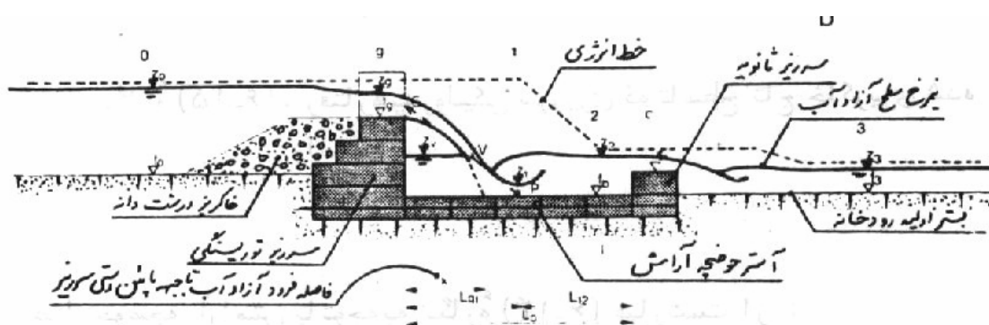
شکل ۳۴: پارامترهای مربوط به تعیین طول حوضچه آرامش (جوان و همکاران، ۱۳۶۹)
