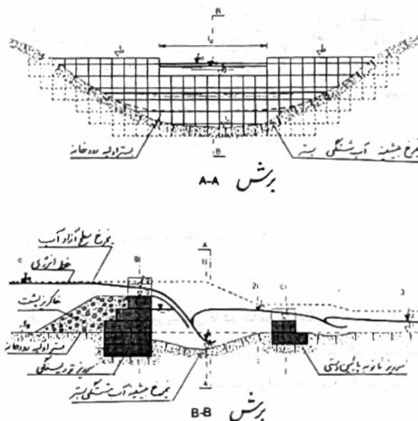
شکل شماره ۲۷ - سرریز توریسنگی قائم با سرریز ثانویه و حوضچه آرامش بی‌آستر (جوان و همکاران ، ۱۳۶۹)
