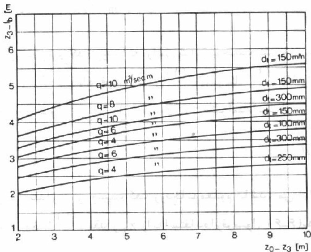
شکل ۳۳: تغییرات عمق آب شستگی بنا بر فرمول شوکلیچ (جوان و همکاران، ۱۳۶۹)
