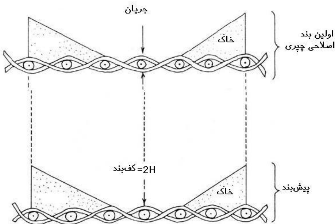
شکل شماره ۵ - تصویر اولین بند اصلاحی چپری همراه با پیش‌بند ( Geyik ، ۱۹۸۶ )
