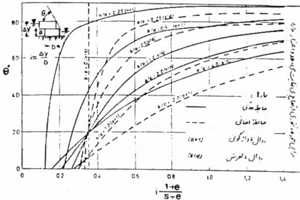
شکل شماره ۲۴ - پایداری تورینگهای پلکانی (جوان و همکاران، ۱۳۷۹)
