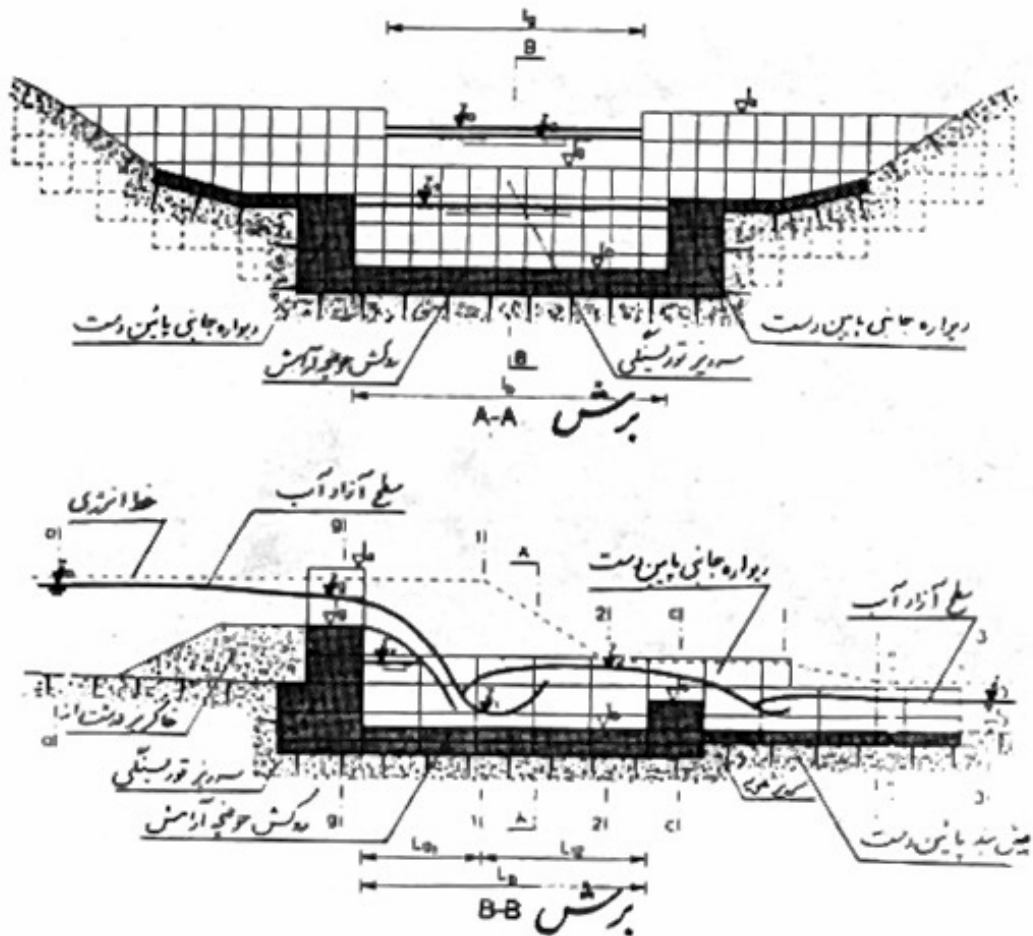
شکل ۲۸ - سرریز توریسنگی قائم با حوضچه آرامش آستردهار همسطح با بستر رودخانه (جوان و همکاران، ۱۳۶۹)
