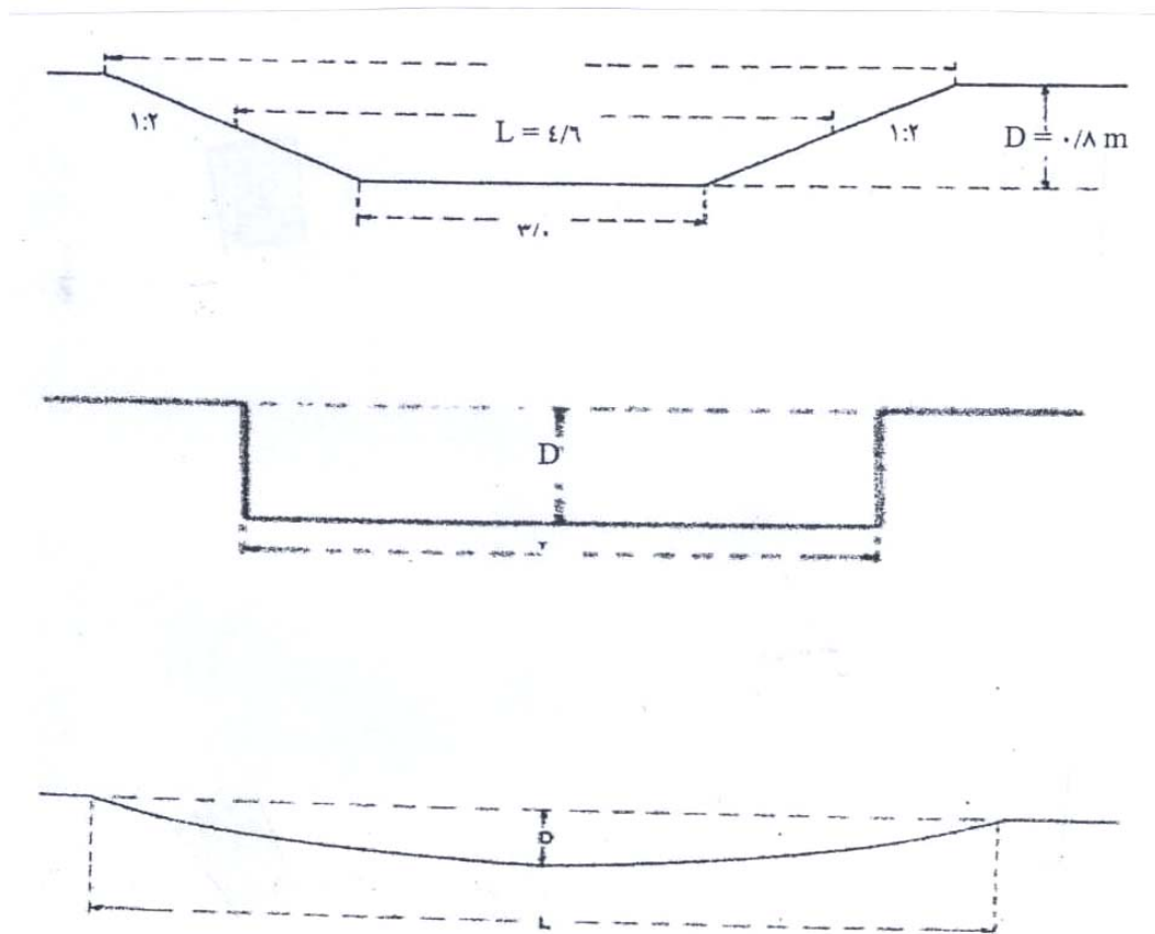
شکل شماره ۲۵ - شکل های معمولی سرریز مورد استفاده در بند اصلاحی (Geyik, ۱۹۸۶)
