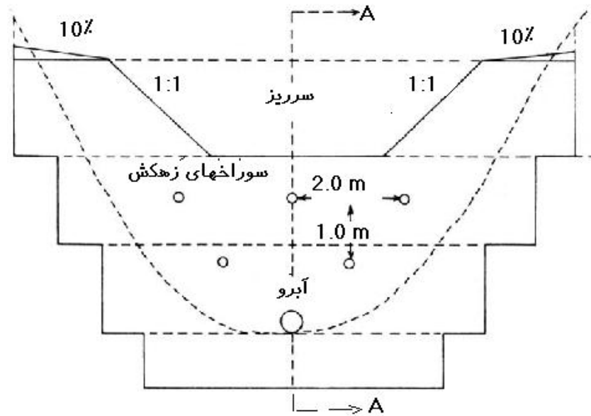
شکل شماره ۱۴ - نمای جلوی اولین بند اصلاحی سنگ و سیمانی (Geyik ، ۱۹۸۶)
