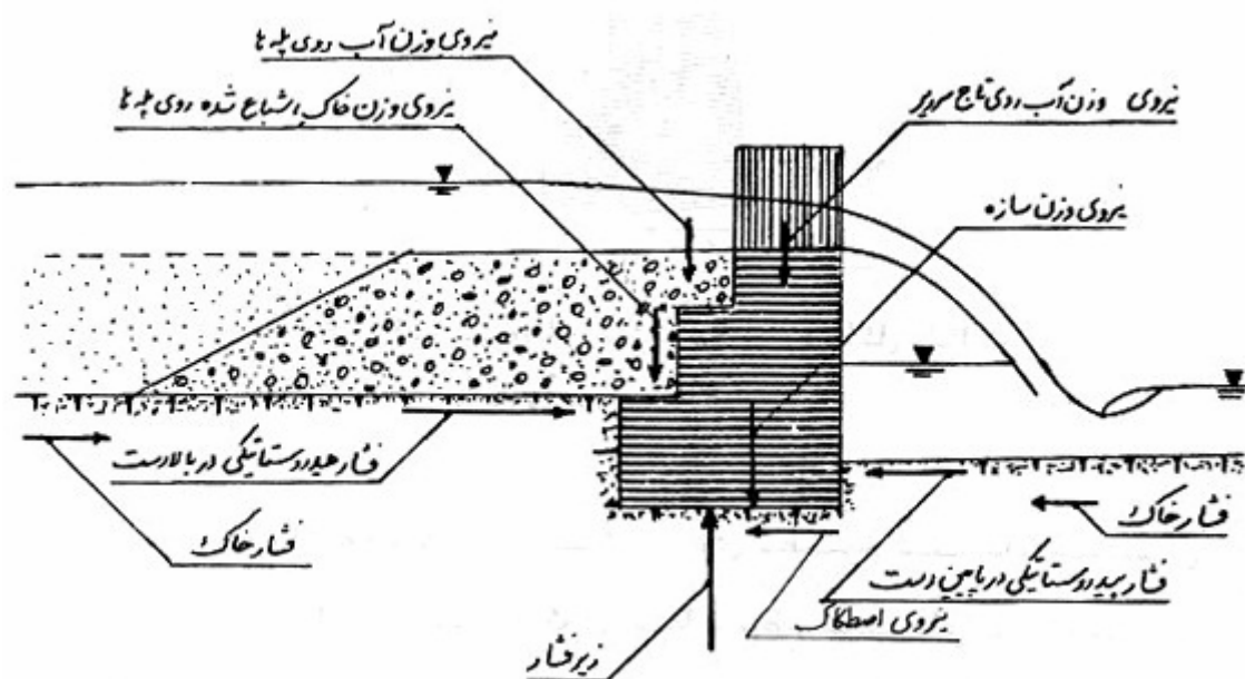
شکل شماره ۲۱- نیروهای وارده بر یک سرریز توریسنگی (جوان و همکاران ، ۱۳۶۹)
