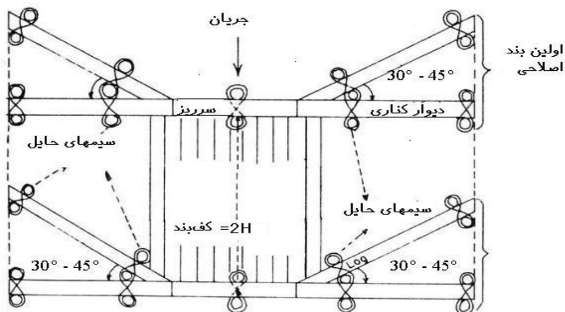
شکل شماره ۶ - تصویر اولین بند اصلاحی الواری همراه با پیش‌بند (Geyik، ۱۹۸۶)
