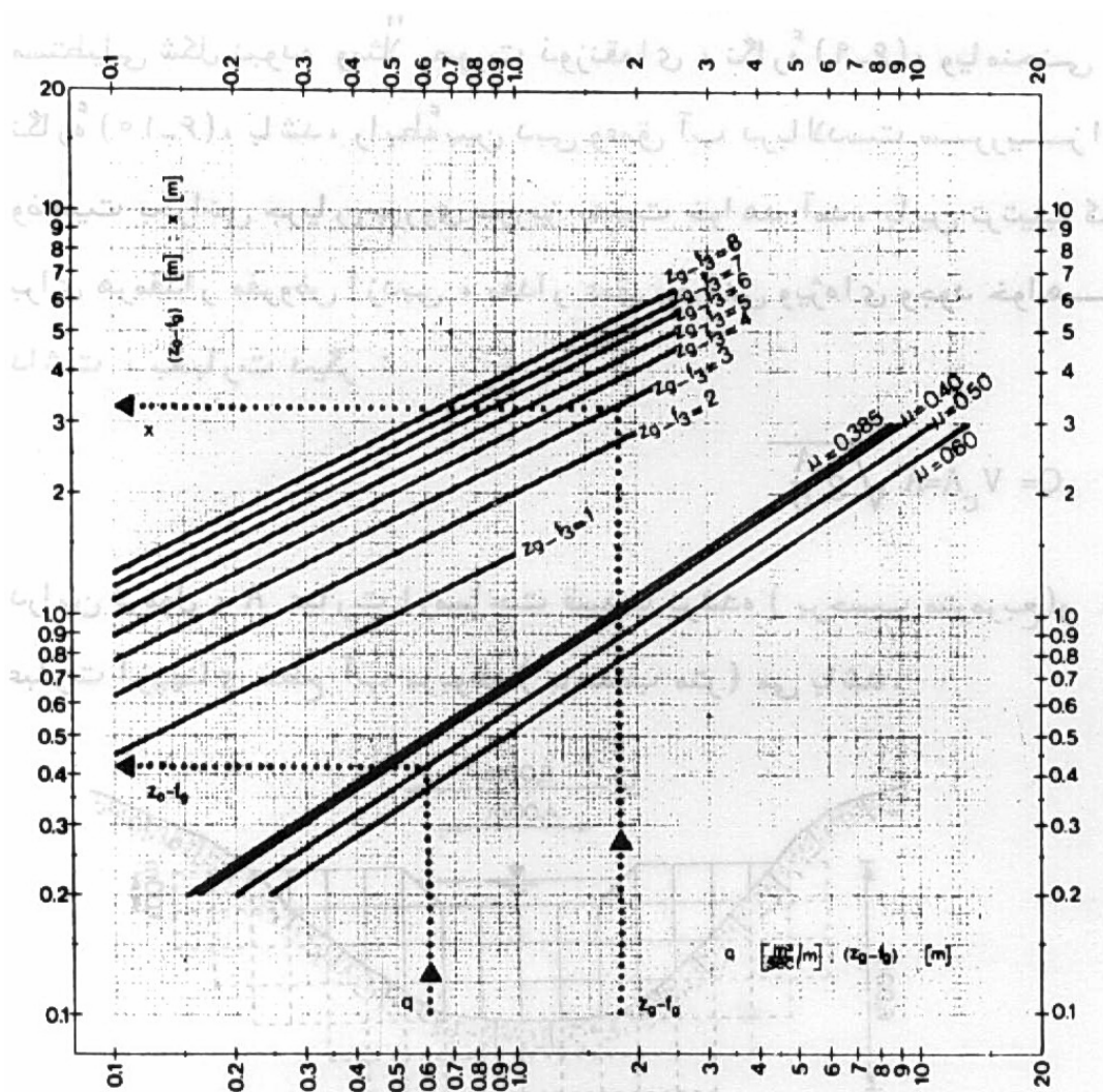
شکل ۳۰ - نمودار (Z_0 - f_g) در طراحی تاج سرریزهای توریسنگی و طراحی حوضچه آرامش
