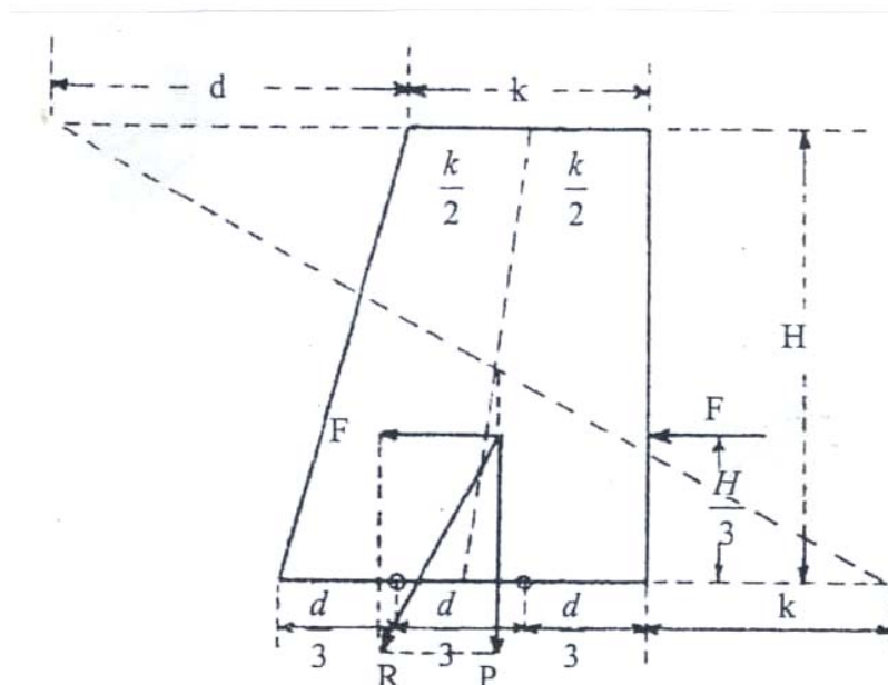
شکل شماره ۲۰- کنترل پایداری بندهای وزن و حجمی با روش گرافیکی - نیروی برآیند R باید از \frac{1}{3} وسطی قاعده بگذرد (Geyik، ۱۹۸۶)
