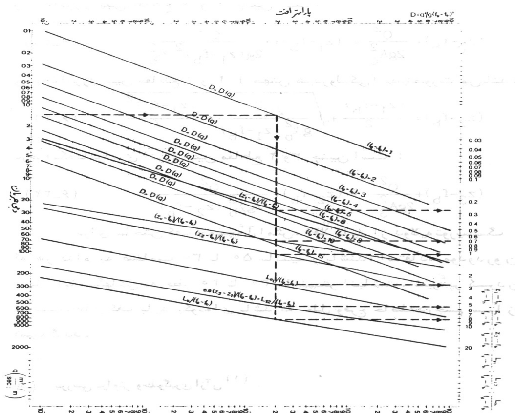
شکل ۳۷ - نمودار تعیین ابعاد حوضچه آرامش سرریزهای توربینی بر حسب پارامتر افت D (جوان و همکاران ، ۱۳۶۹)
