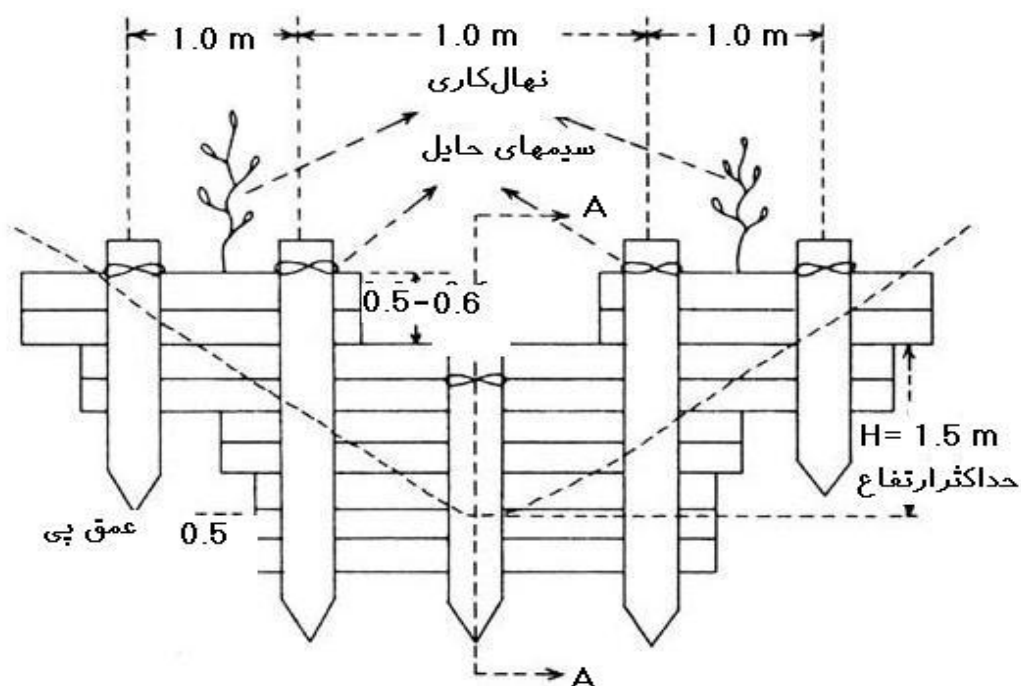
شکل شماره ۷ - نمای جلوی اولین بند اصلاحی الواری (Geyik، ۱۹۸۶)
