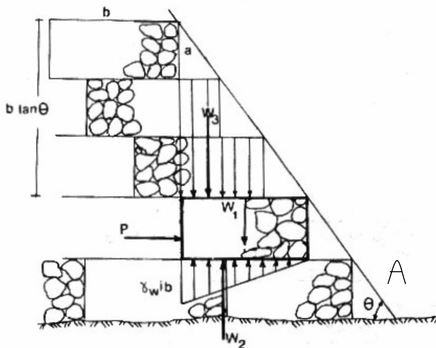
شکل شماره ۲۳- نیروهای وارده بر پیکر آزاد یک واحد توريسنگی در یک سازه پلکانی (جوان و همکاران ، ۱۳۷۹)
