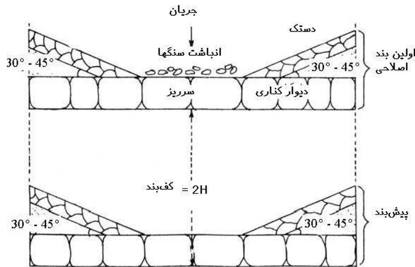
شکل شماره ۱۳ - تصویر اولین بند اصلاحی قلوه سنگی با پیش بند (Geyik ، ۱۹۸۶)
