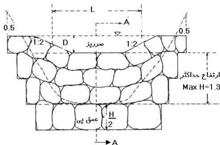
شکل شماره ۱۲ - مقطع اولین بند اصلاحی قلوه‌سنگی با پیش‌بند (Geyik، ۱۹۸۶)
