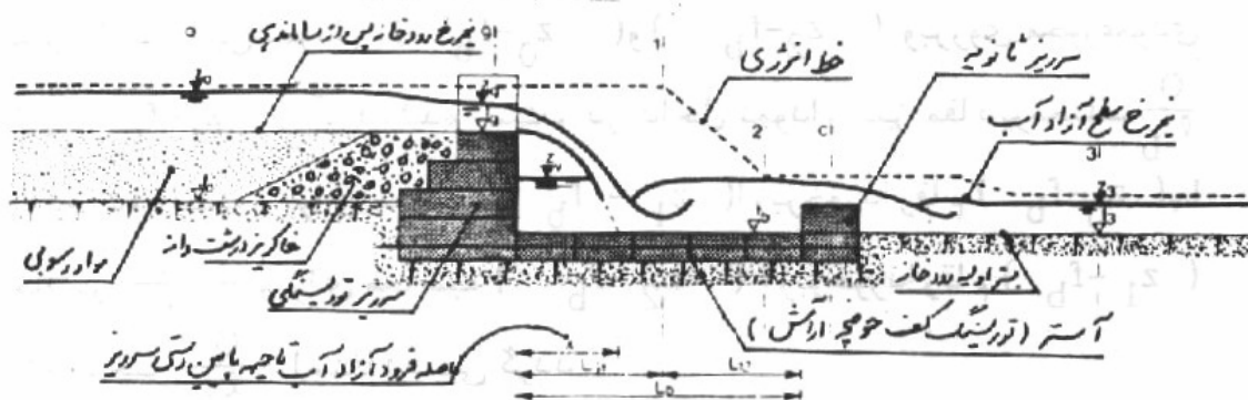
شکل ۳۵: رفتار هیدرولیکی سرریزی تا سطح تاج خاکریزی شده (جوان و همکاران، ۱۳۶۹)
