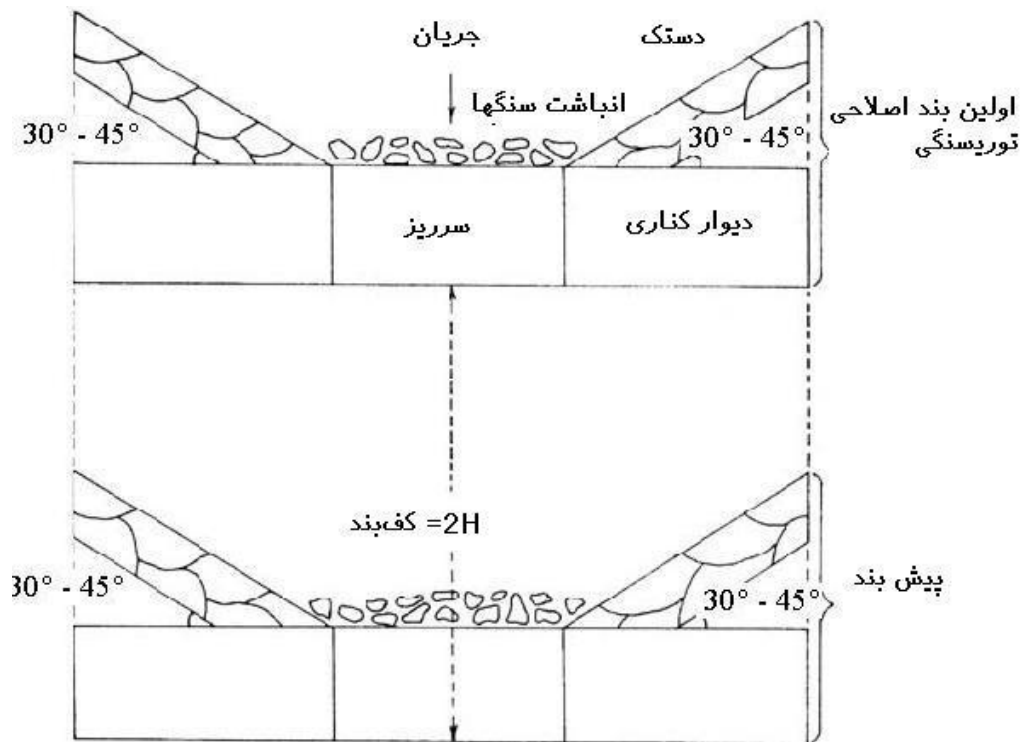
شکل شماره ۱۹ - تصویر اولین بند اصلاحی توریسنگی با پیش بند (Geyik ، ۱۹۸۶)
