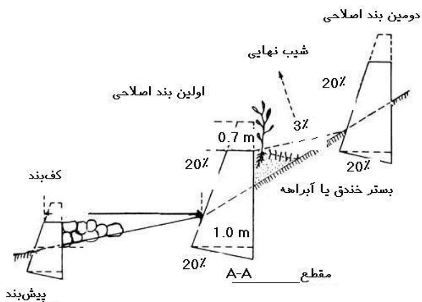
شکل شماره ۱۰- مقطع اولین بند اصلاحی خشکچین همراه با پیش بند (Geyik، ۱۹۸۶)
