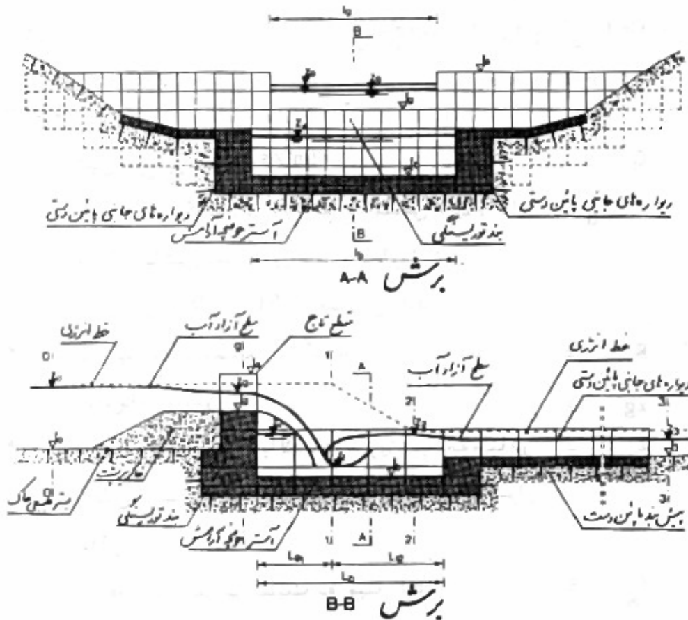
شکل ۲۹ - بند توریسنگی قائم با حوضچه آرامش آسترदार (عمیق تر از کف رودخانه) با کنترل جهش هیدرولیکی با ایجاد پله انتهایی
