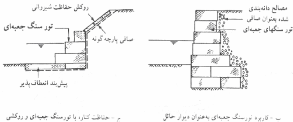
شکل ۲۳ - دیوارهای گابیونی
