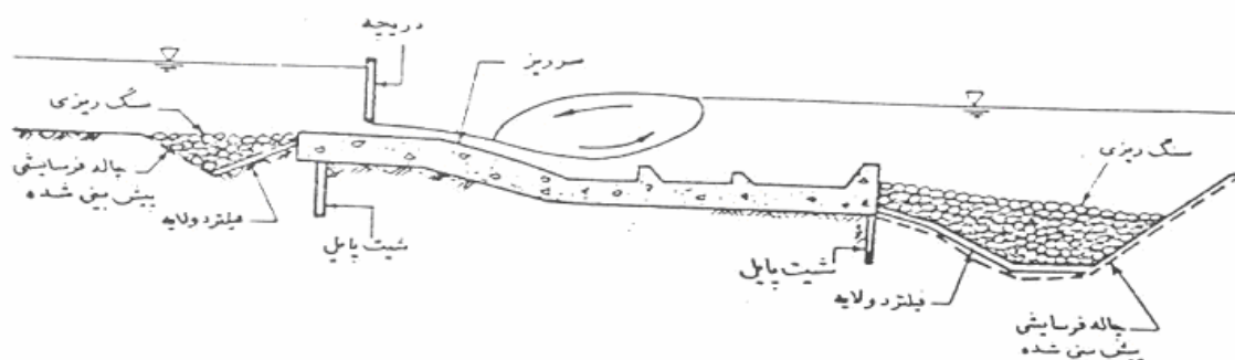
ب - نمونه‌ای از تلفیق سازه صلب (سرریز و حوضچه آرامش) و سازه انعطاف پذیر برای تثبیت بستر
