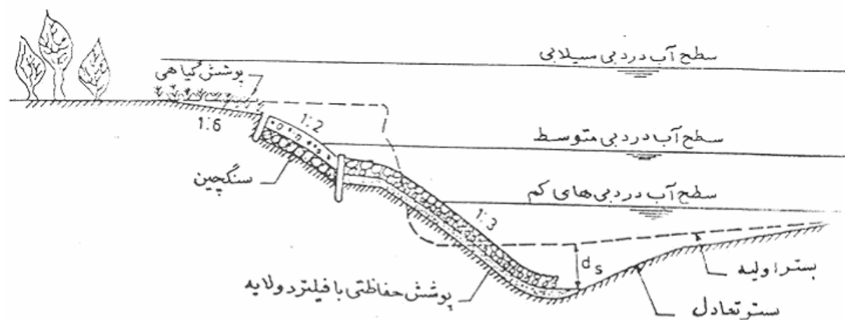
الف - مقطع پوشش حفاظتی سنگچین فیلتردار برای کنترل فرسایش کناره‌ها
