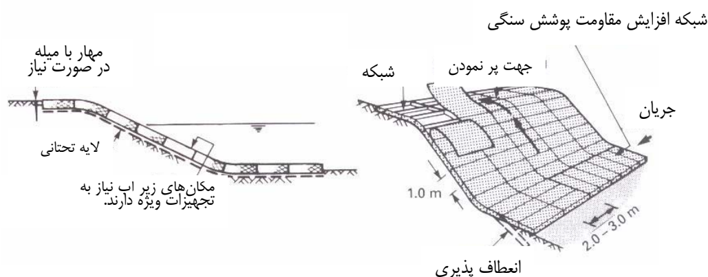
شکل (۱۸) - پوشش تشک گابیونی
