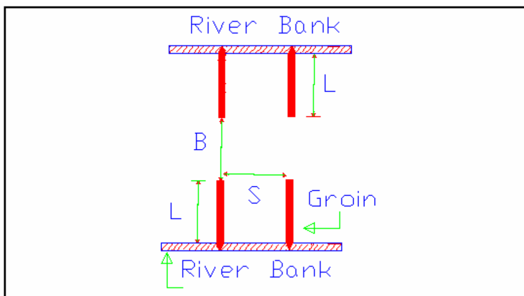
شکل (۴) - نمایش پارامترهای عرض کنترل شده رودخانه (B)، طول آبشکن (L) و فاصله آبشکن‌ها (S) براساس توصیه‌های ممک و ولوسنی
