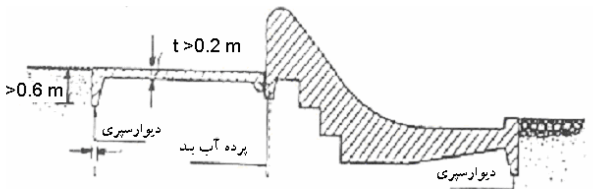
شکل ۳۳- دیواره‌های سپری بالادست و پایین‌دست در شیب‌شکن‌ها
