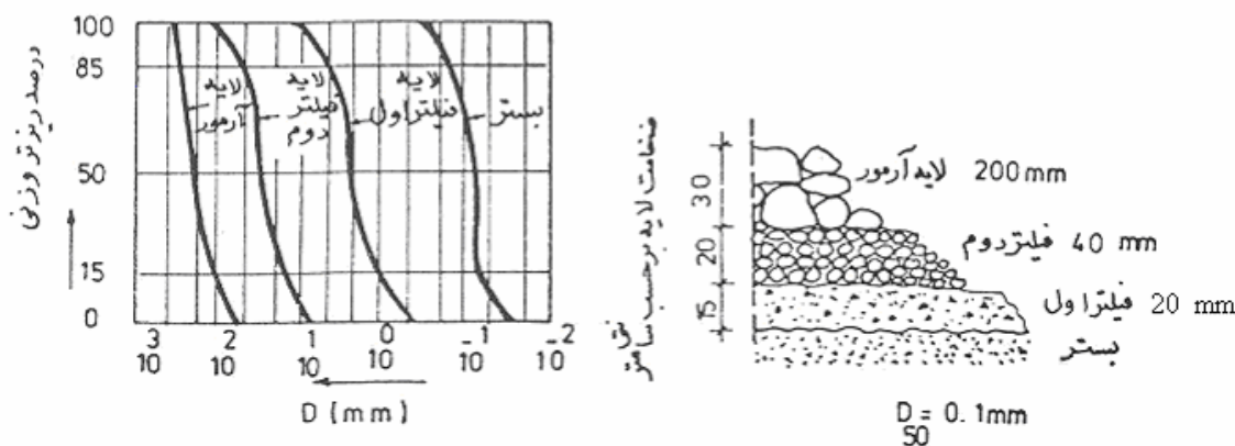
ب - مشخصات دانه‌بندی بستر و لایه فیلتر و آرمور پوشش حفاظتی
