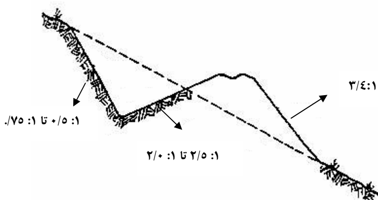
شکل شماره ۳ - نمونه‌ای از بانکت با شیب عرضی به طرف داخل
