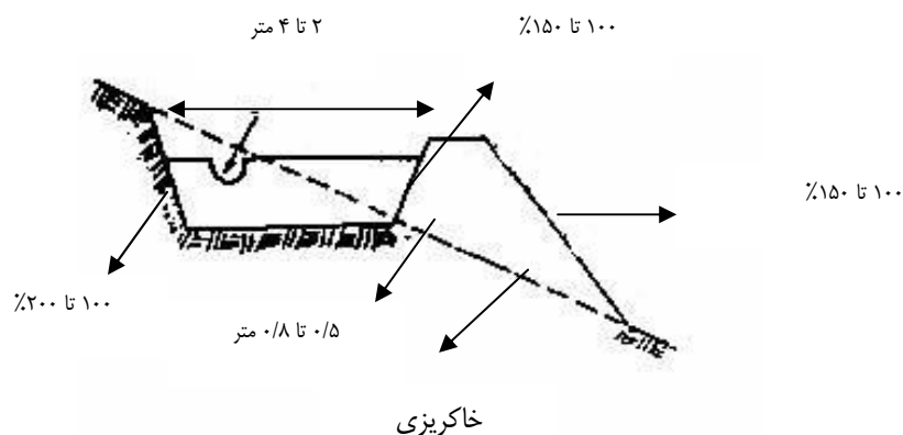
شکل شماره ۶ - یک بانکت دوزنقه‌ای شکل
