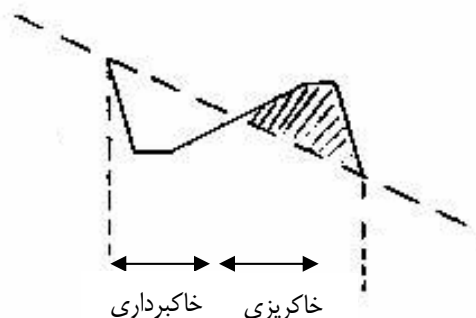
شکل شماره ۱۵- روش دو خطی پیاده نمودن بانکت‌ها
