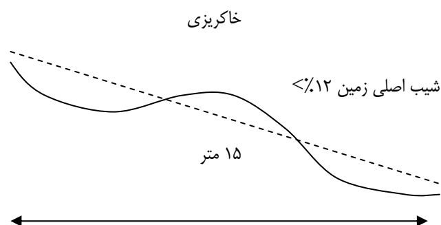
شکل شماره ۱۲ - نمای یک بانکت با انحنای سه گانه (مانگام)
