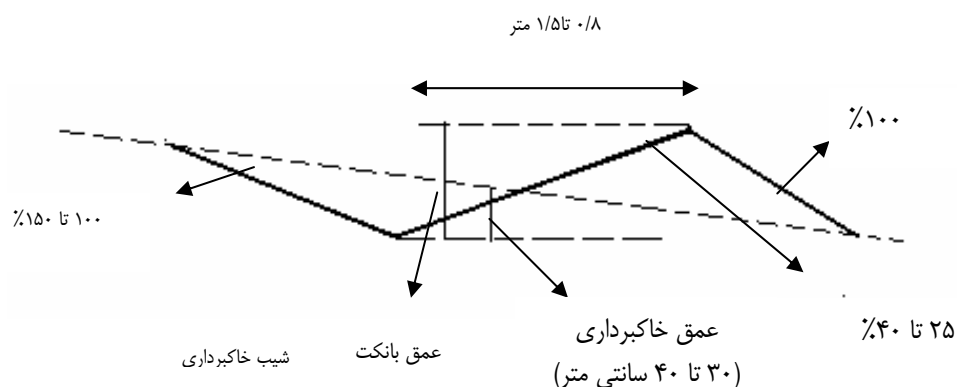
شکل شماره ۵ - بانکت مثلثی شکل
