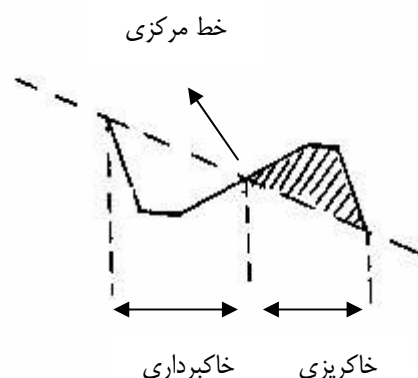
شکل شماره ۱۴ - روش سه خطی پیاده نمودن بانکت ها
