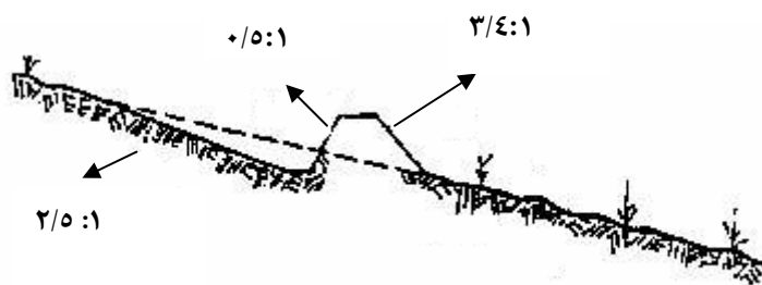
شکل شماره ۲ - بانکت با شیب عرضی به طرف خارج
