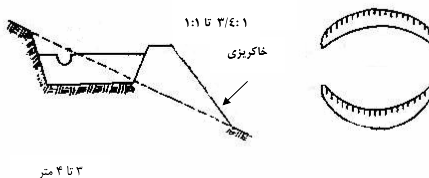
شکل شماره ۴- بانکت بدون شیب عرضی
