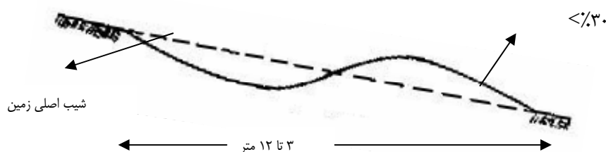
شکل شماره ۷ - نمونه ای از بانکت انحنایی شکل
