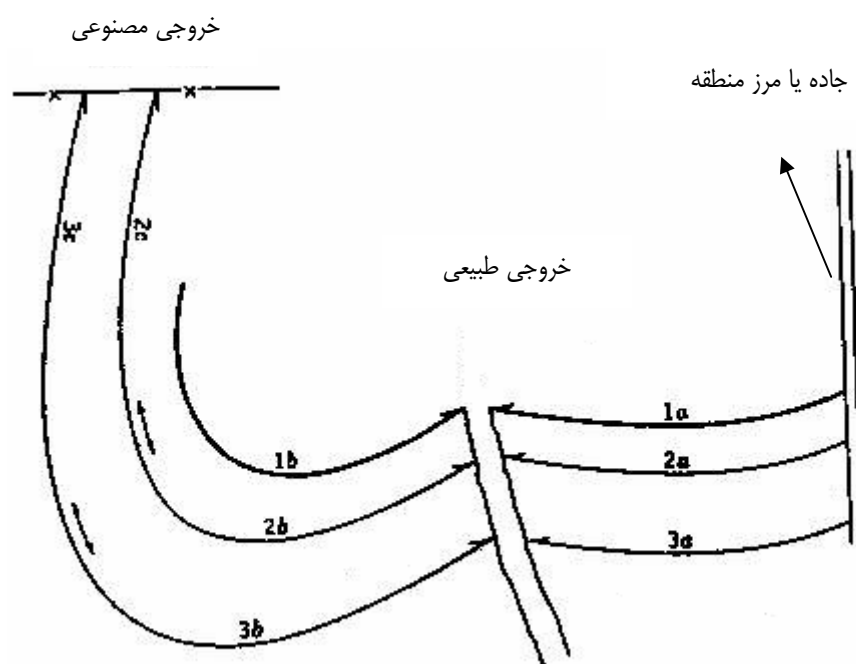
شکل شماره ۱۳ - طرح ریزی خروجی در یک سیستم بانکت بندی
