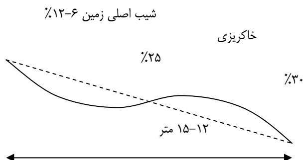
شکل شماره ۱۰ - نمای یک بانکت نیکولز
