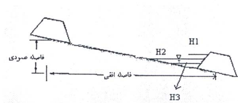
شکل شماره ۱۷ - پارامترهای مربوط به ارتفاع سکوهای خاکی
