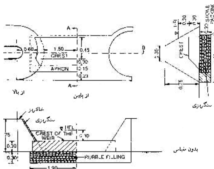
شکل شماره ۸ سربز بدون مانع
