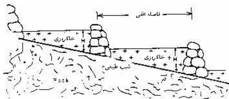
شکل شماره ۳ سکو بندی سنگی با شیب مصنوعی (و خاکریزی)
