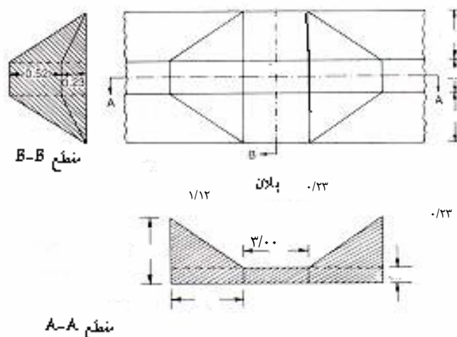
شکل شماره ۷ سرریز پله‌ای (موقتی)
