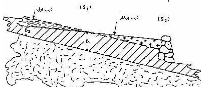
شکل شماره ۱ سکو بندی سنگی با شیب طبیعی (شیب پایدار در اثر فرسایش)
