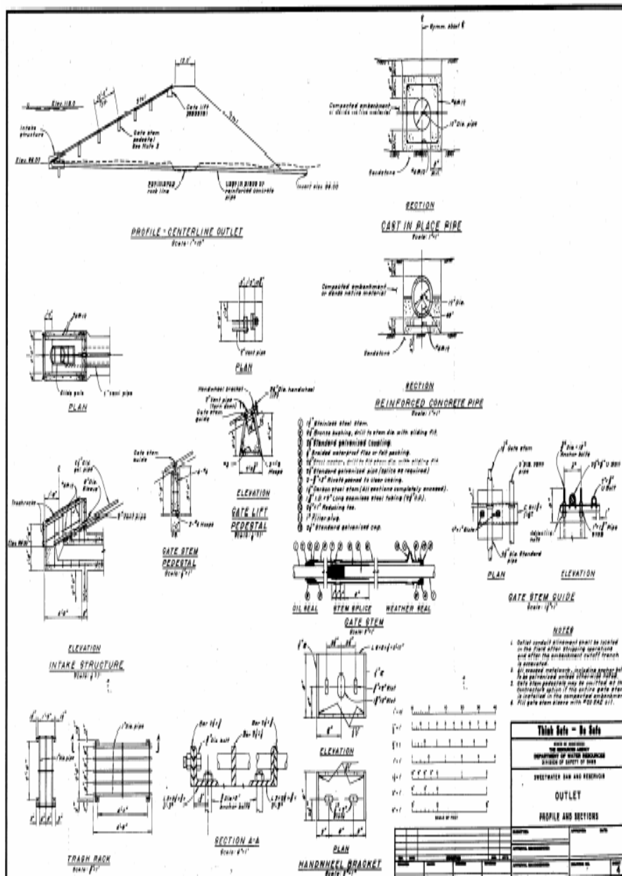
شکل شماره ۴۱ - نقشه الکویی پروفیل و مقاطع مجرای خروجی
