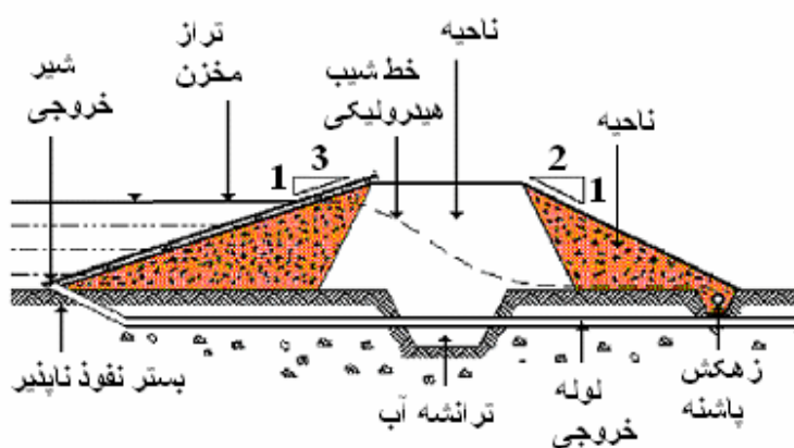
شکل شماره ۱۸ - پلان و مقطع تبیین سدهای کوچک زراعتی
