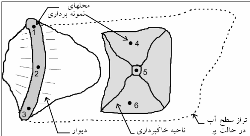
شکل شماره ۲۵ - نقشه پلان سد خاکی و دریچه آن و محل نمونه برداری
