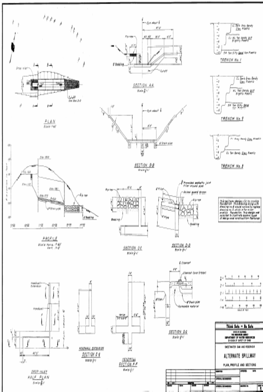
شکل شماره ۴۲ - نقشه الکویی پلان، پروفیل و مقاطع نوع دیگری از سرریز
