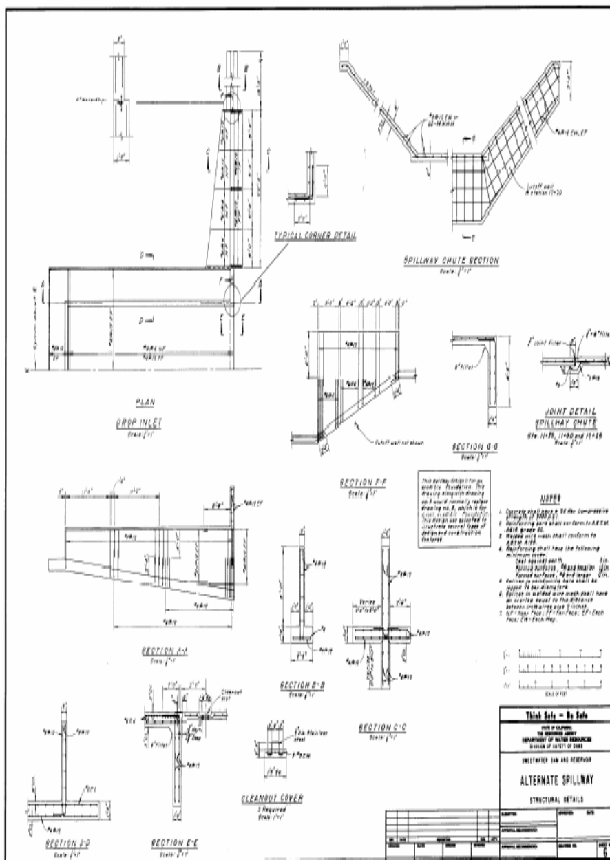
شکل شماره ۴۳ - جزئیات سازه ای سرریز
