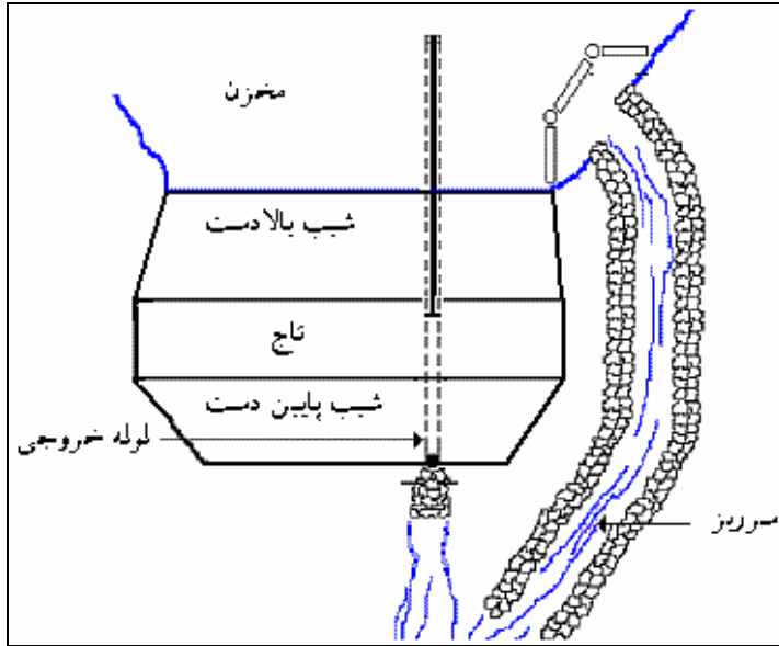
شکل شماره ۲۴- پلان تیپ یک سد زراعتی
