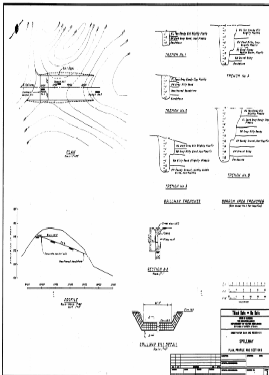
شکل شماره ۴۰ - نقشه الگویی پلان و مقاطع سرریز
