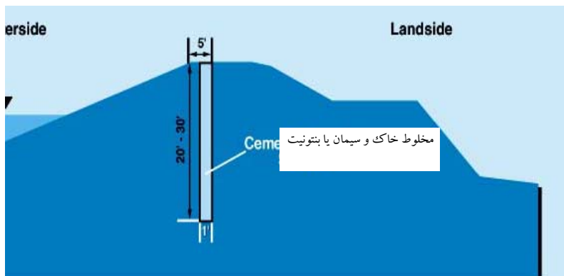
شکل شماره ۴ - یکی از روش‌های آب‌بندی گورهاها (دیواره آب‌بند) (اقتباس از سایت رودخانه‌ها و سواحل ایران)
