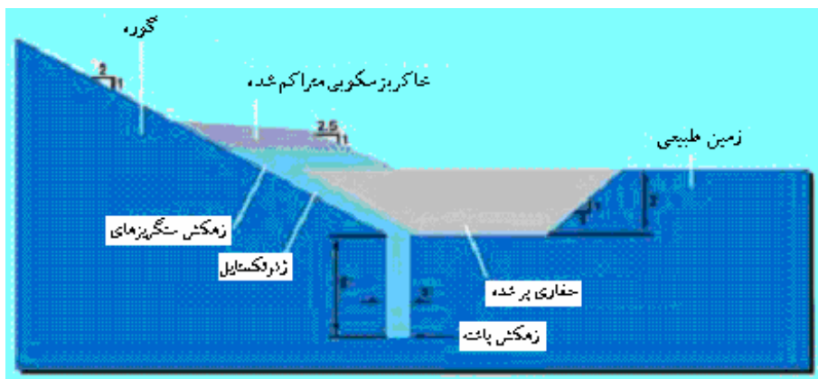
شکل شماره ۵ - زهکش پاشنه گورهاها (اقتباس از سایت رودخانه‌ها و سواحل ایران)
