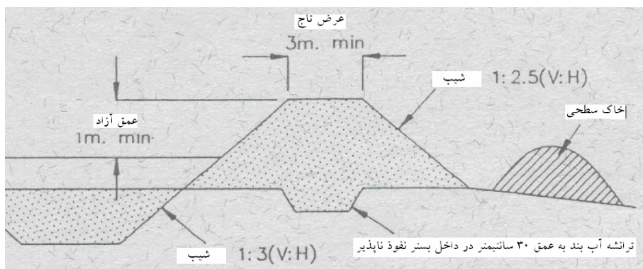
شکل شماره ۱۹ - مقطع عرضی سد کوچک زراعتی و دریاچه آن
