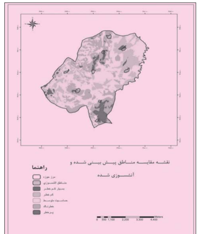
شکل ۵- نقشه مقایسه مناطق پیش بینی شده و آتش‌سوزی شده در منطقه سراوان
