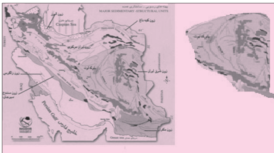
شکل ۴- وضعیت زمین‌شناسی منطقه مورد مطالعه
