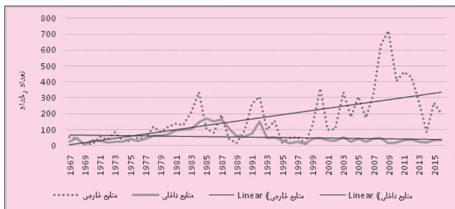
شکل ۴- روند تغییرات رخداد گرد و غبار از منابع داخلی و خارجی
